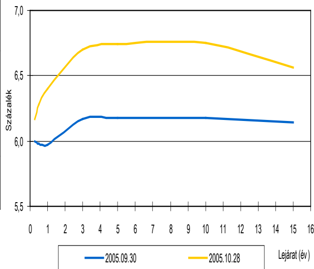
Referenciahozam-görbe
