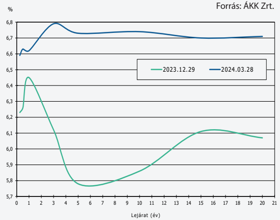
Referenciahozam-görbe
