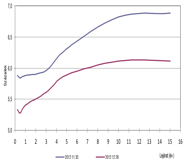
Referenciahozam-görbe
